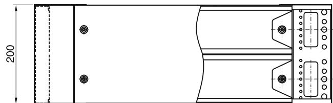
Maßbild Sockel 200 mm hoch
